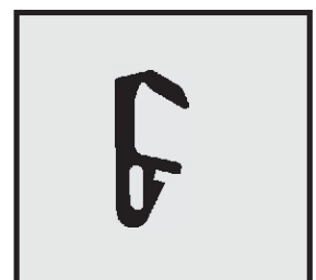
Profil-Nr. SD 2041 Farbe schwarz Material EPDM
