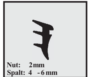
Profil-Nr. SD 2036 Farbe schwarz Material EPDM
