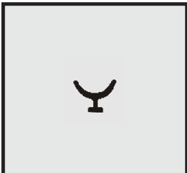
Profil-Nr. SD 5129 Farbe weiß Material TPE
