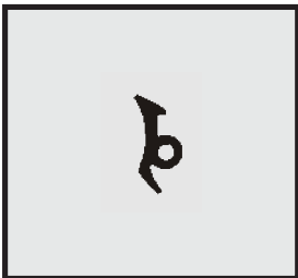
Profil-Nr. SD 5084 Farbe schwarz Material TPE
