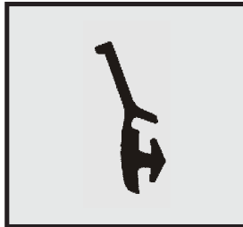
Profil-Nr. SD 5258 Farbe schwarz Material TPE
